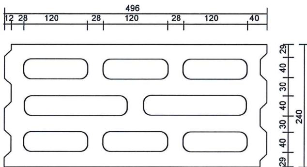
Bild 5 HBL 2-0,8 16DF
