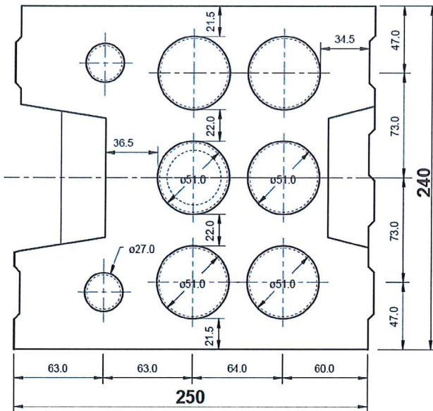
Bild 3 KSL 12 8DF
