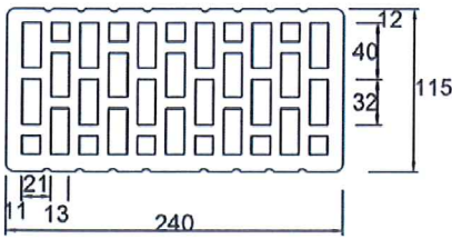
Bild 1 HLZ 12 2DF
